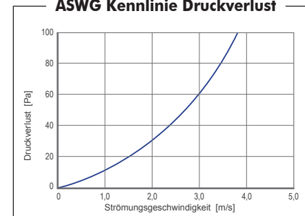
ASWG Kennlinie Druckverlust
